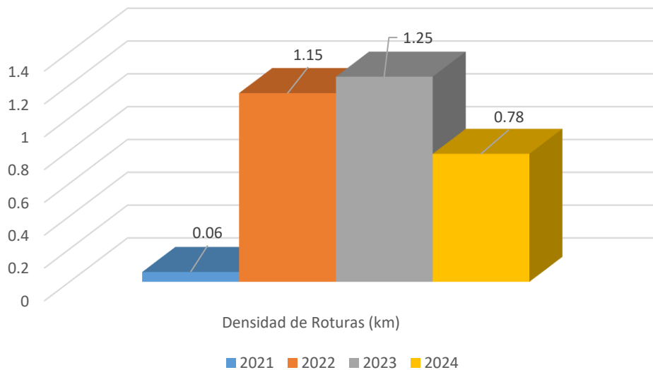
Ilustración 13: Densidad de Roturas de Redes de Agua Potable (Km) a nivel EPS
